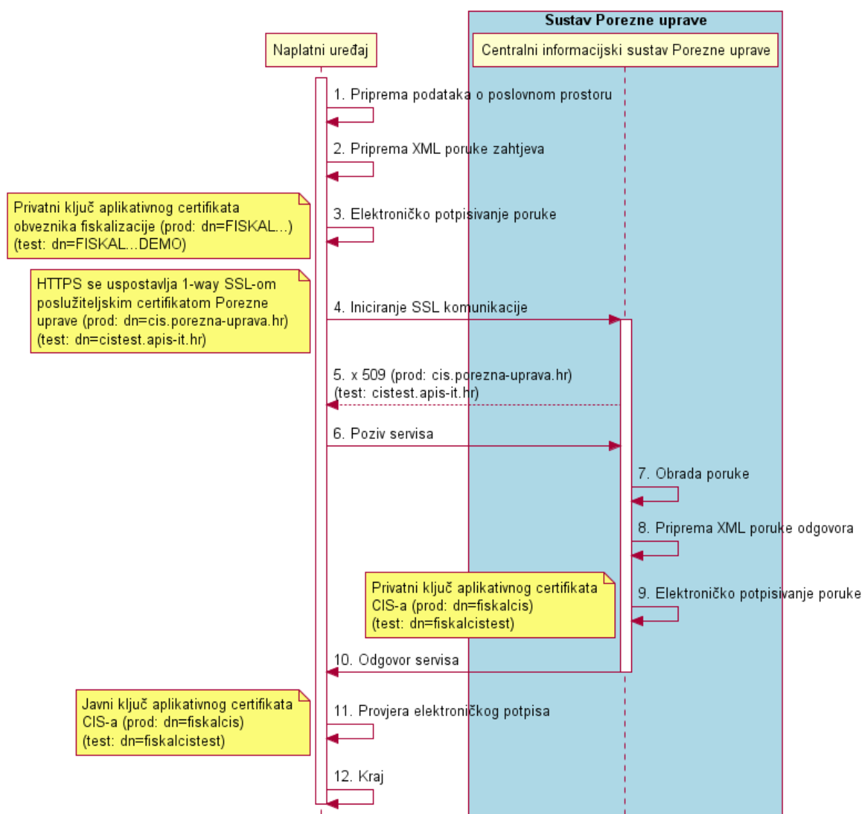
Slika 5. Slijedni dijagram procesa za slanje podataka o poslovnom prostoru
