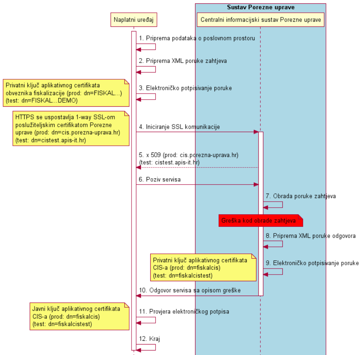
Slika 6. Slijedni dijagram procesa za slanje podataka o poslovnom prostoru u slučaju greške
