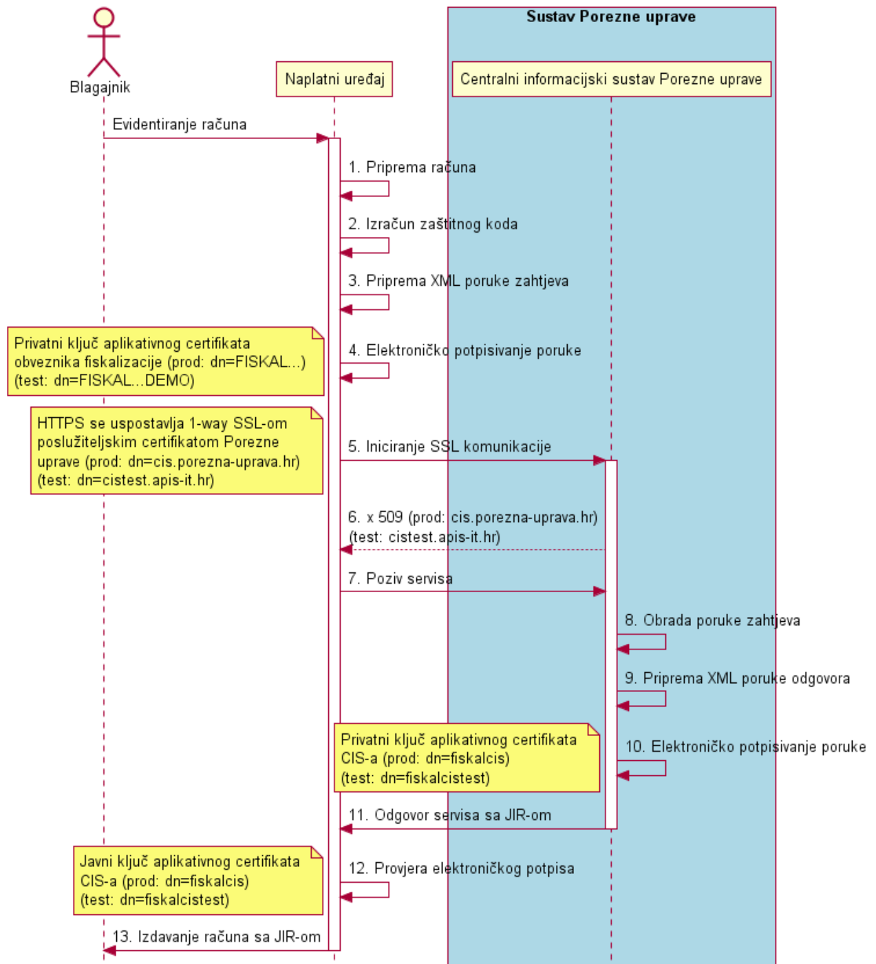
Slika 1. Slijedni dijagram procesa za slanje računa
