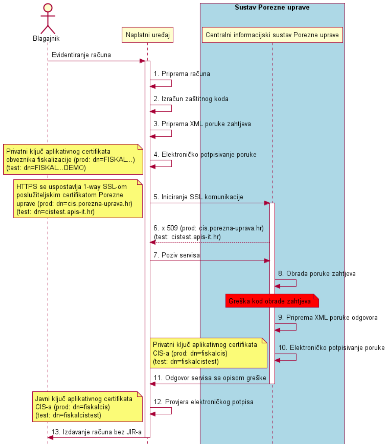
Slika 2. Slijedni dijagram procesa za slanje računa u slučaju greške
